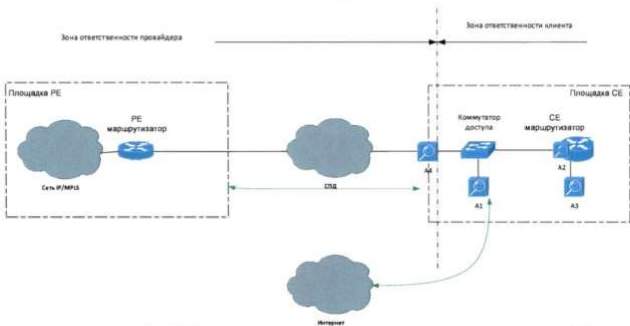
Рис.1. Типовые схемы подключения зондов на площадке типа CE
